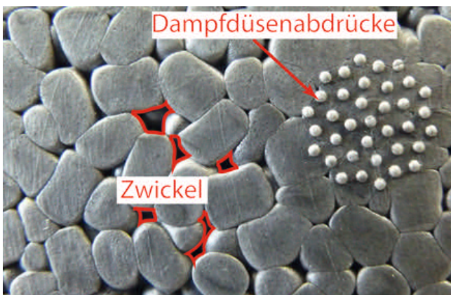
Bild 1. Charakteristische Oberfläche eines Partikelschaumformteils aus EPP mit einer Dichte von ca. 50 kg/m 3 (Bild: NMB)
